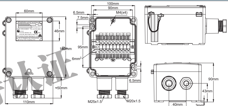
带接线柱的示例
